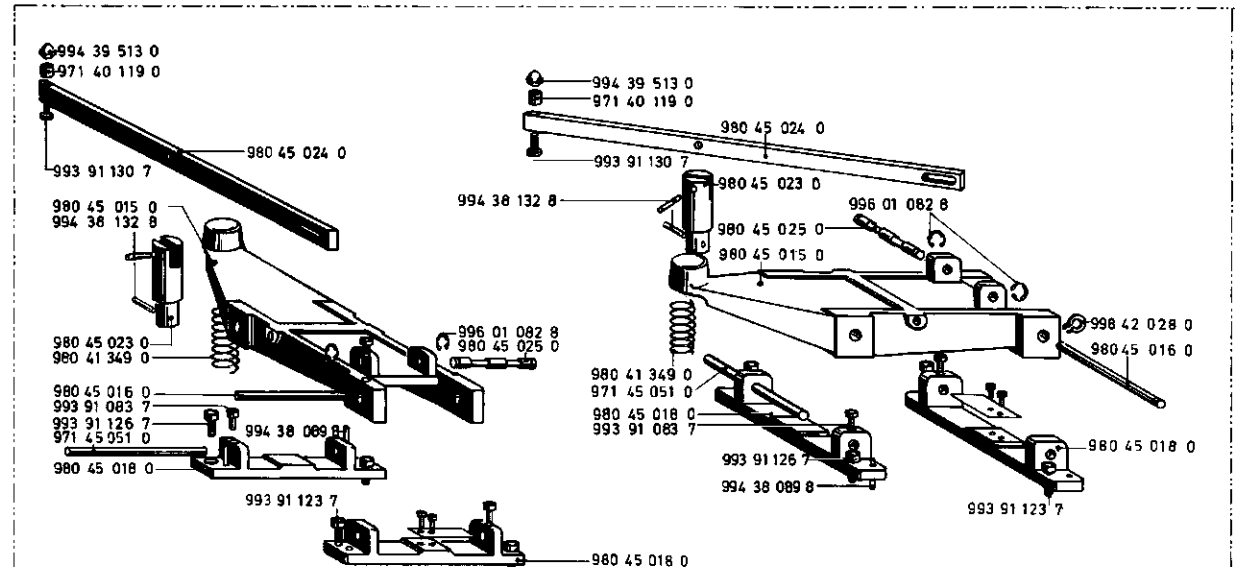
Segmentsatz Kpl. 971 45 804 4 nur 1/4 gezeichnet
