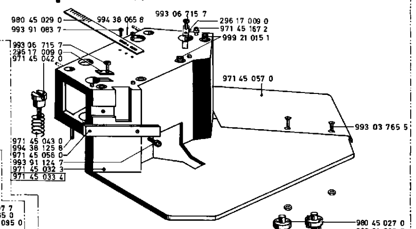
Segmentsatz Kpl. 971 45 804 4 nur 1/4 gezeichnet
